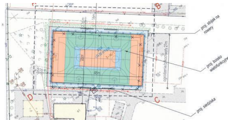
Projekt planowanego boiska wielofunkcyjnego w Gorenii Dużym
